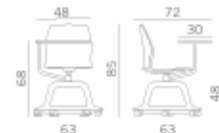
Sedia girevole c/tavoletta scrittoio ruotabile a 360° Swivel chair w/360° rotating writing tablet
