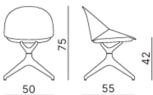
Telaio girevole piramidale 4 piedi nylon Pyramidal swivel nylon 4-leg base
