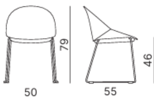
Telaio slitta in acciaio Steel sled frame
