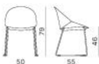
Telaio slitta in acciaio Steel sled frame
